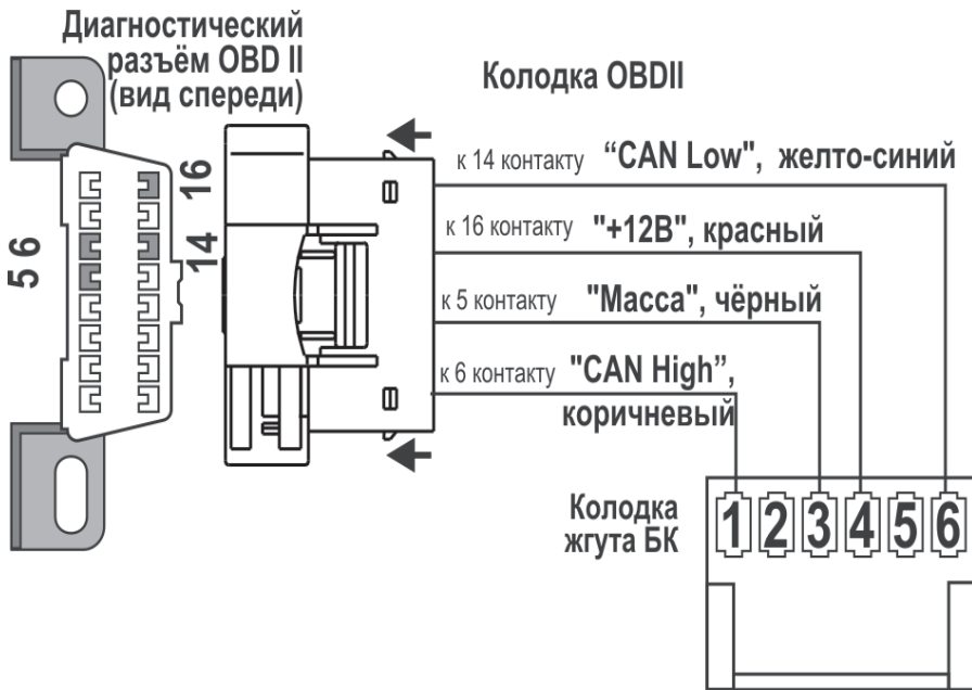
Рис.2 Схема подключения БК "ШТАТ Х1"
